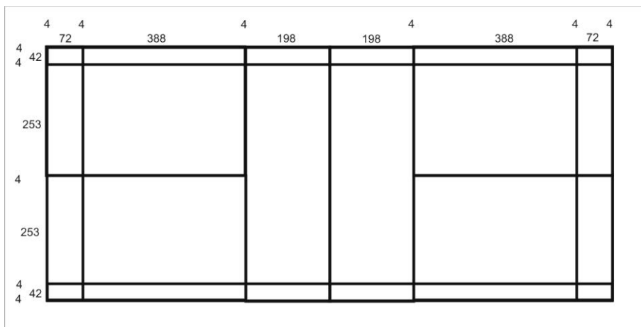
PIIRROS A. Yhdistetty kaksin- ja nelinpelikenttä. Mitat senttimetrejä.
